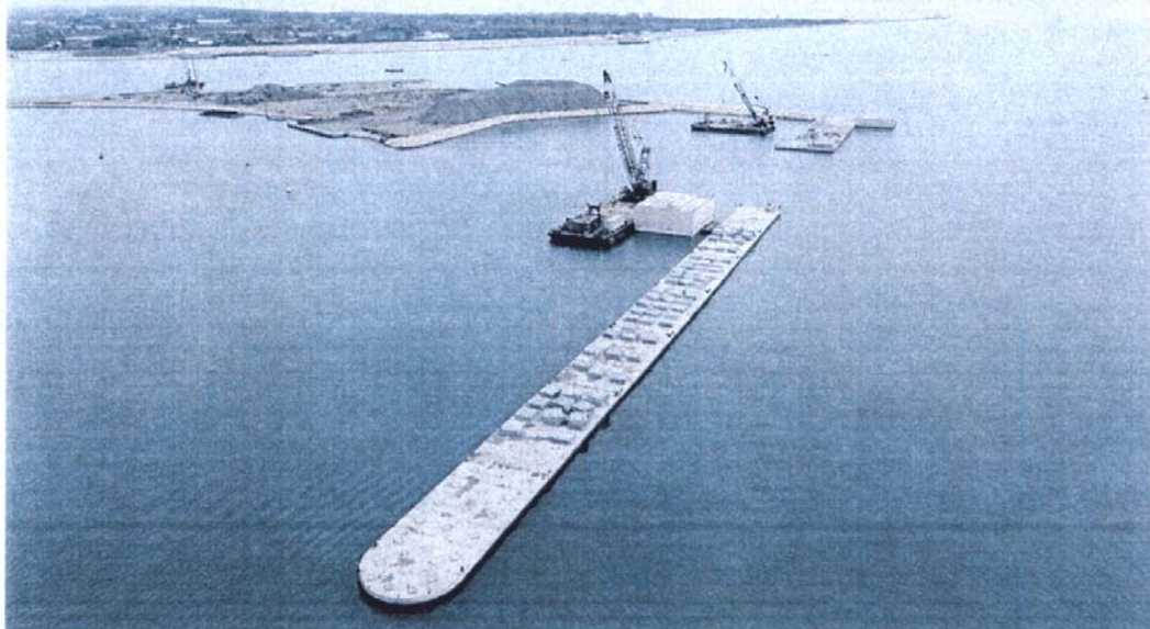
Bocca di Lido - S. Nicolò: la spalla nord di S. Nicolò, in via di definizione. In primo piano i cassoni prefabbricati già posati.
