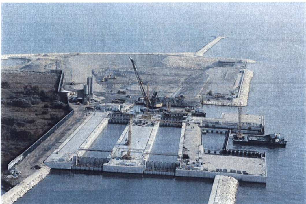
Bocca di Chioggia : veduta generale delle conche di navigazione e della spalla nord della barriera. Sullo sfondo il porto rifugio lato mare messo all'asclutto.
