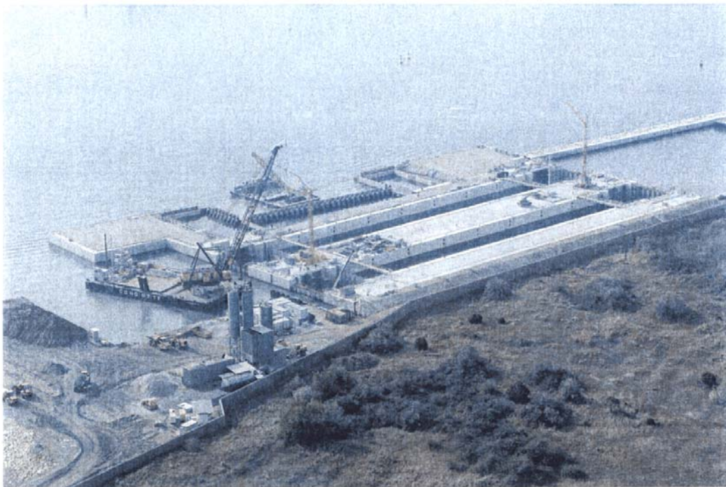
Bocca di Chioggia : veduta lato Cà Roman delle conche di navigazione (In primo piano) e delle strutture della spalla nord in via di realizzazione.
