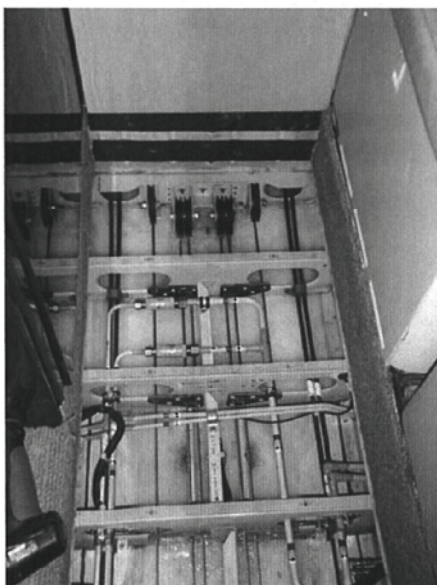
P180 marche di immatricolazione N140SL: prove sul sistema di cavi e pulegge della trasmissione dei comandi.
