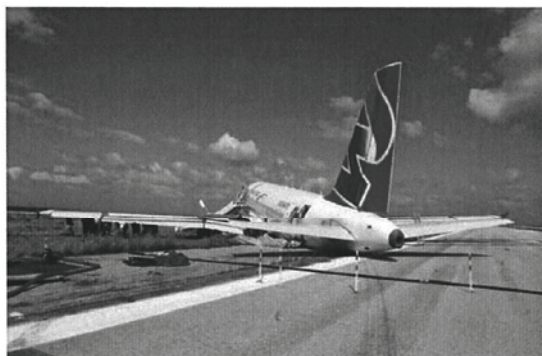
A319 EI-EDM: alcune immagini riprese nel punto di arresto del velivolo.
