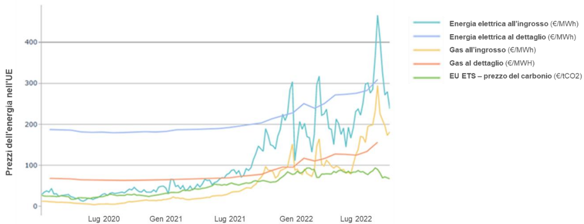
Figura 1. Prezzi all'ingrosso e al dettaglio di gas ed energia elettrica e prezzi del carbonio nell'UE. Fonti: Platts, VaasaETT
