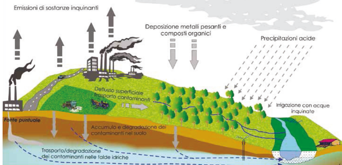
Figura 8.09 Schema della contaminazione diffusa Fonte ISPRA
