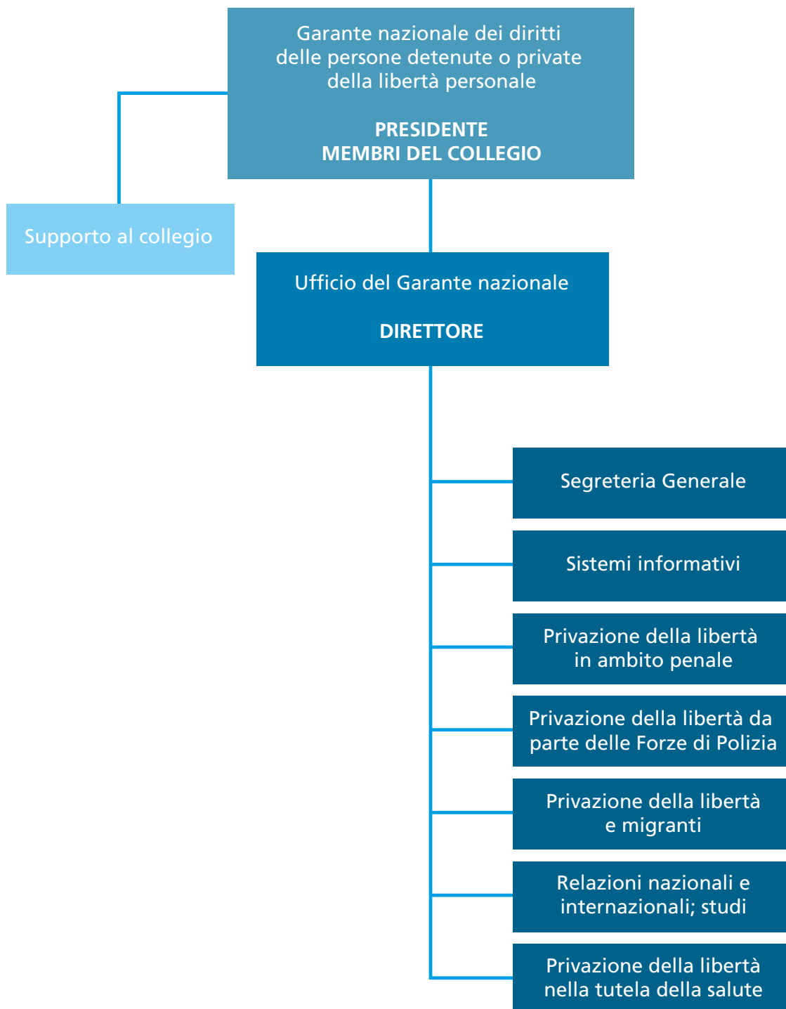
Grafico 7.1 - Organigramma dell'Ufficio
