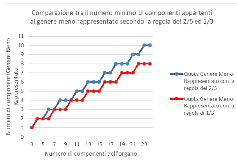
Figura 3 – Analisi di sensitività
