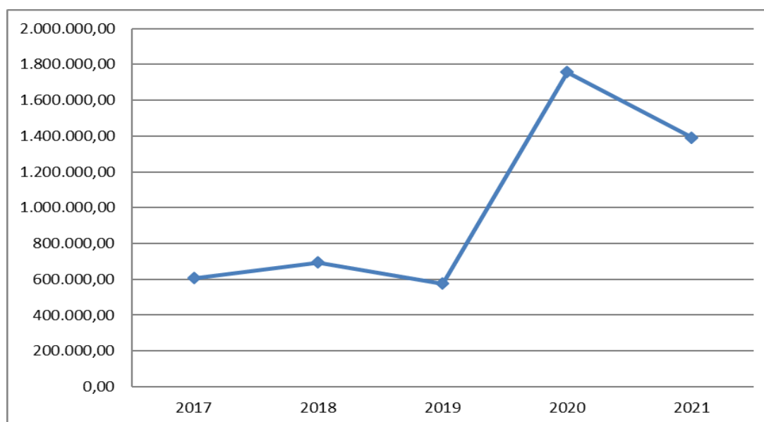
Grafico n. 8: Andamento dello "avanzo di amministrazione non vincolato" relativo alle "Strutture di Ricerca" negli anni compresi tra il 2017 e il 2021
