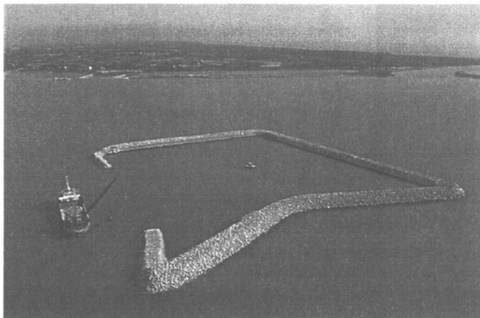
Bocca di Lido - Isola tra S. Nicolò e Treporti 1 ^ fase
