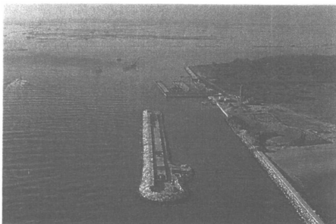
Bocca di Chioggia – Porto rifugio – Scogliera sud Conche per piccole imbarcazioni
