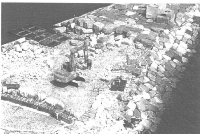
Bocca di Malamocco- Diga foranea. Mezzi in opera.
