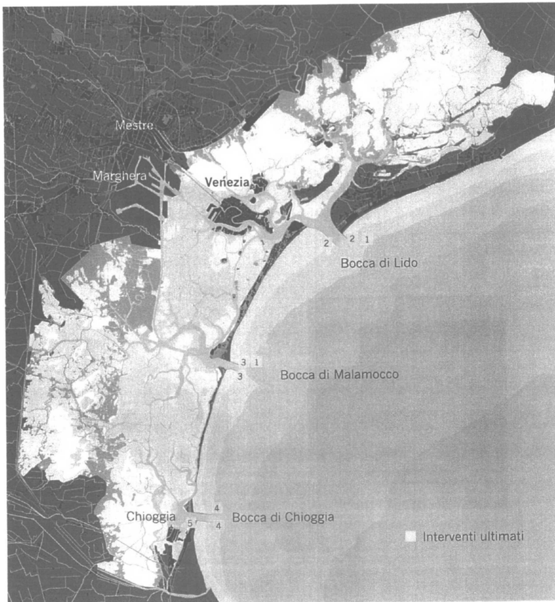
RISTRUTTURAZIONE DEI MOLII FORANEI ATTIVITA' ULTIME (nessuna attività è attualmente in corso)
