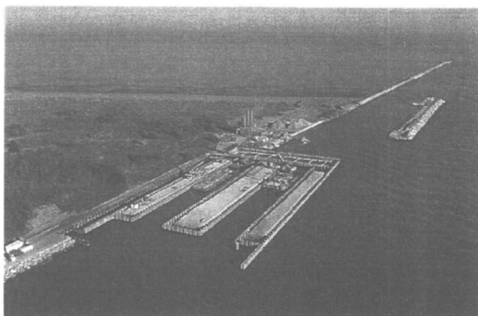
Bocca di Chioggia – Conche di navigazione. Fasi di realizzazione delle conche.
