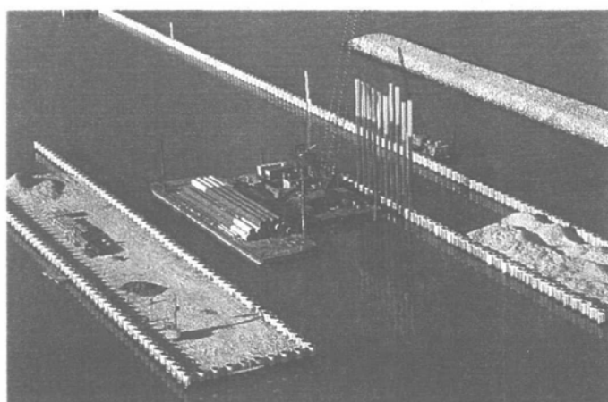
Bocca di Malamocco – Conca di navigazione – camera di conca. Realizzazione riempimenti.
