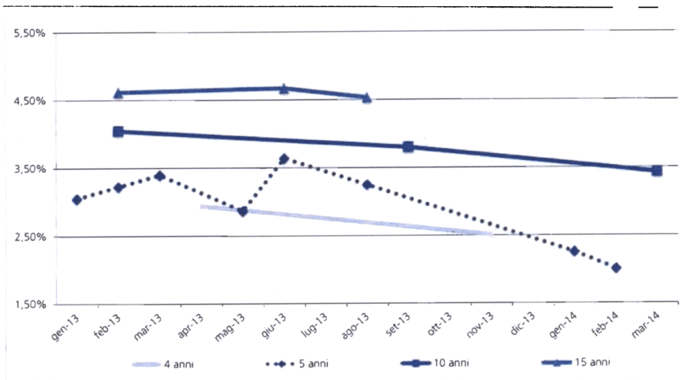
Figura 3-7 : Rendimenti lordi all'emissione del BTPEi e del BTP Italia
