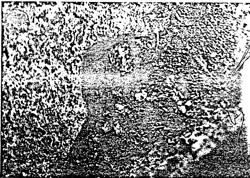
FOTO 20.- Incrostazione di bitume rinvenuta al bordo della scarpa sinistra dell'On.MORO, con visibili sulla superficie alcuni granuli di sabbia. Altro è presente ancora sotto le suole, su oggetti rinvenuti sul pavimento ed altrove all'interno della vettura, sotto i pneumatici della Renault R4.-
