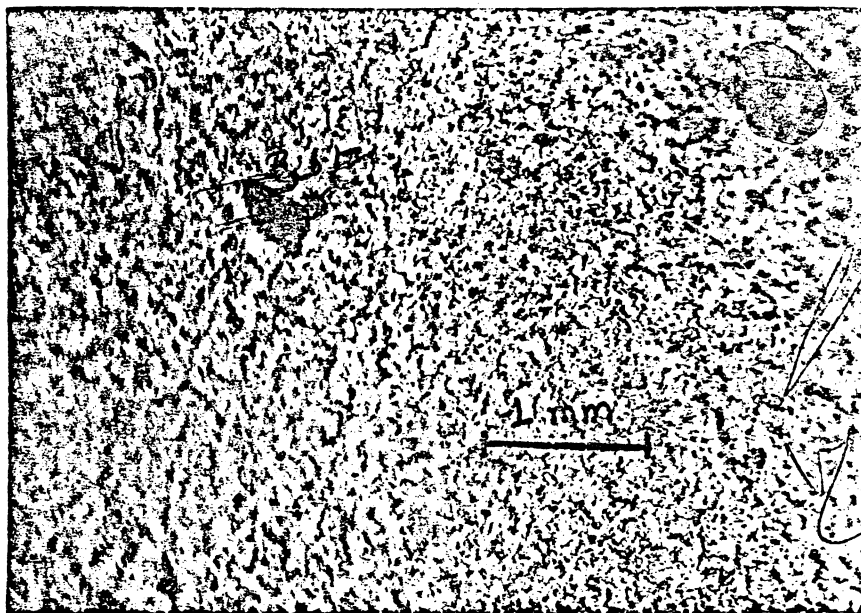
FOTO 15.- Suola delle scarpe indossate dall'On.MORO. E' ben visibile un frammento di mica biotite, affiancato ad altri granuli minerali biancastri. Questo ed altri frammenti di minerali vulcanici presentano caratteri morfoscopici che indicano come hanno subito scarso o nullo trasporto.-
