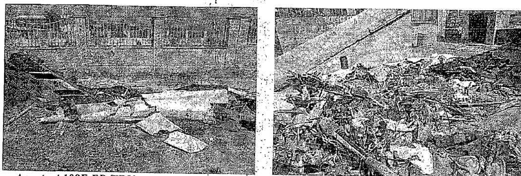
Agusta A109E EP-TRK: trave di coda (foto a sinistra); fusoliera e rotore principale (foto a destra).
